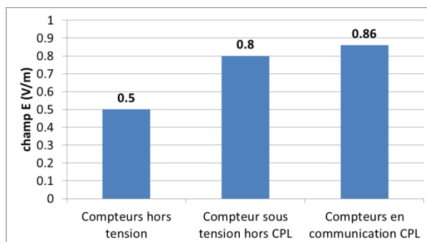
Figure 12 : niveau de champ électrique mesuré dans la bande 1,2 – 100 kHz dans différentes configurations en face du compteur Linky G1.
